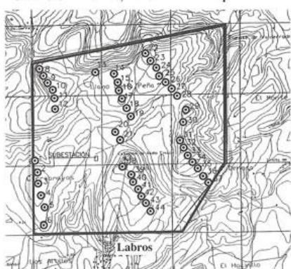
Plano de la disposición prevista por la empresa para instalar sus 44 molinos, con su cerco correspondiente.
